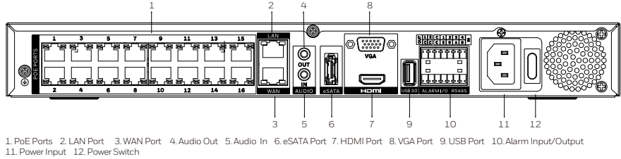
HN351602xxC
