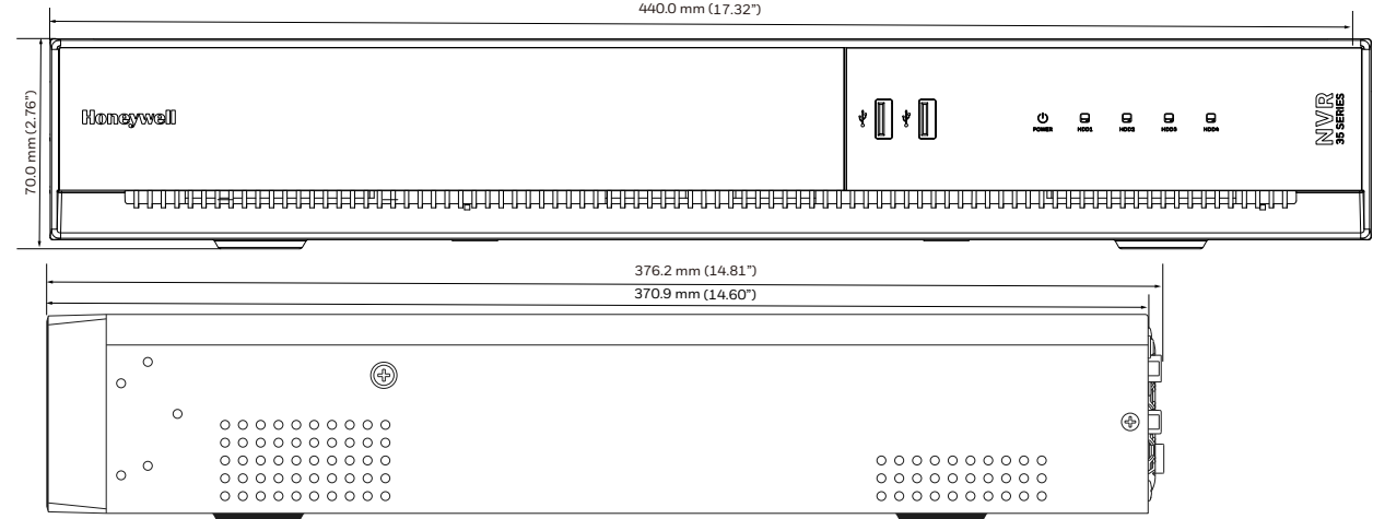
HN351604xxC/HN353204xx
